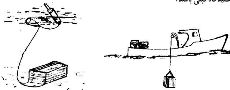
شکل ۴-۷- نصب قفس به صورت منفرد و نحوه بالا کشیدن آن با استفاده از وینچ
