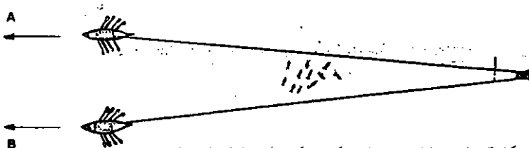
شکل ۴-۵- عملیات صید با تور کششی کیسه‌ای ساحلی با دو قایق
